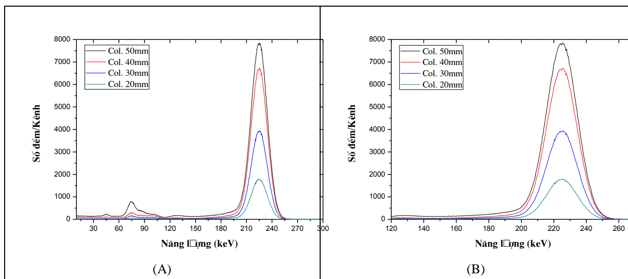
Hình 2. Phổ đáp ứng của đầu dò NaI(Tl) được sử dụng trong nghiên cứu đối với tia gamma năng lượng 224,88 keV cho từng ống chuẩn trực đầu dò (Col.) có đường kính khác nhau được xác định bằng chương trình MCNP5 (A) biểu diễn toàn phổ, (B) biểu diễn trong vùng năng lượng 120-260 keV
